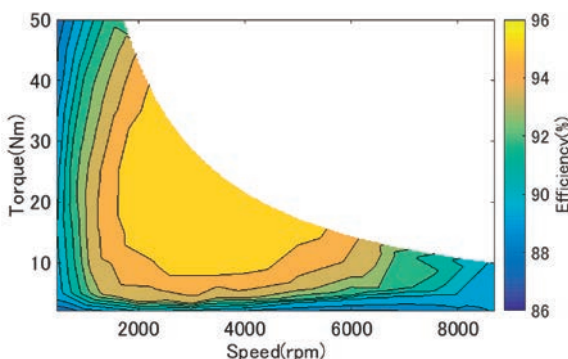
效率图显示例 (MATLAB)
