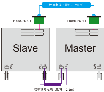
【并联运行系统 4kVA 的实例】
