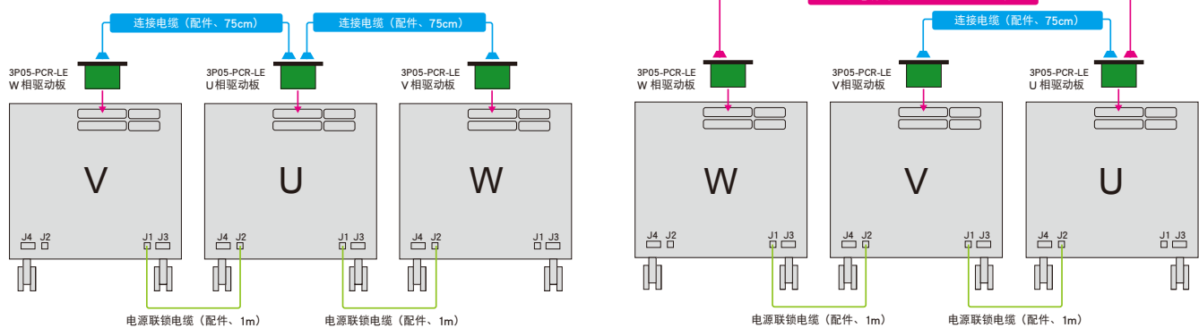
【PCR2000LE 三相系统 6kVA 的实例】
