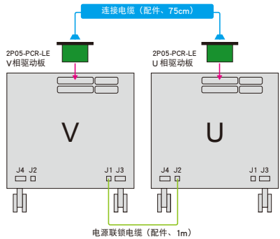
【单相 3 线系统 4kVA 的实例】
