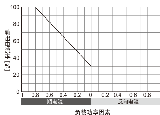
■ 负载功率因素－额定输出电流特性
