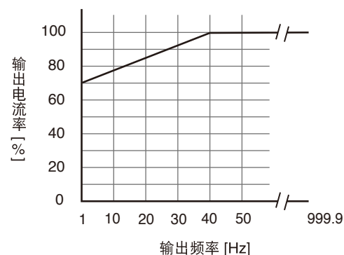
■ 输出频率－额定输出电流特性
