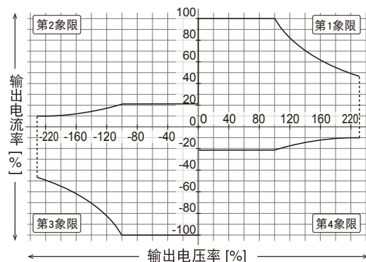
■ 输出电压率－额定输出电流特性 (DC 模式)
