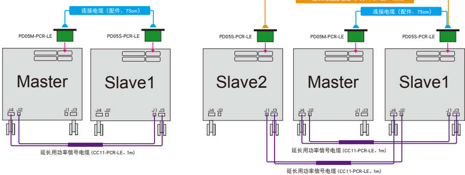
【并联运行系统 6kVA 的实例】
